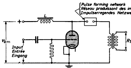
Trigger circuit Circuit déclencheur Abzugstromkreis
